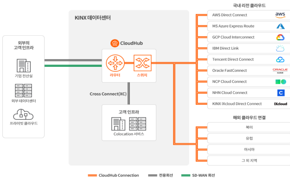
그림39. 케이아이엔엑스 클라우드허브(Cloudhub) 구성도
